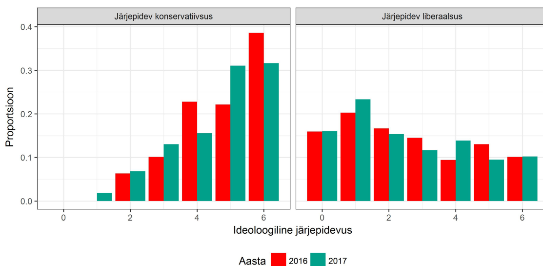
Joonis 9: Liberaalide ja konservatiivide jaotus vastavalt sellele, kui järjepidevalt nad valitud küsimuste puhul vastasid.
